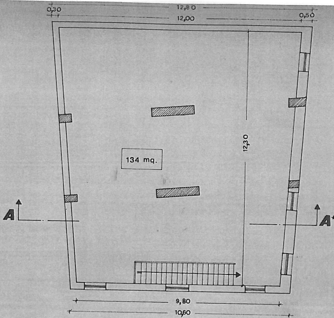
PIANTA PRIMO PIANO
