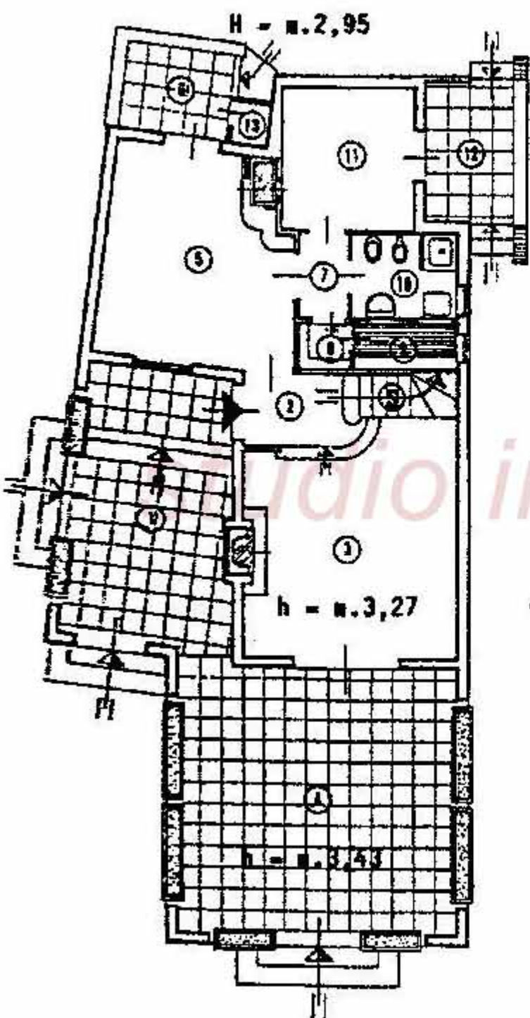
PIANTA A PIANO TERRA
